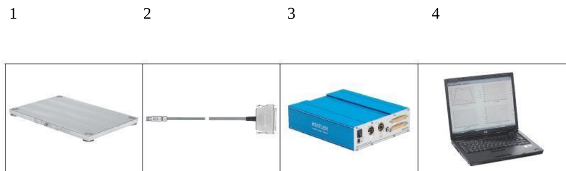
Obr. 1 Merací reťazec systému KISTLER
